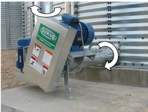
SWEEPWAY (DK) Lodret tømmesystem - (UK) Vertical unloading system - (DE) Vertikal Entladesystem.
