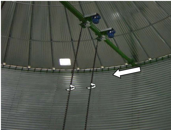
FASTIR (DK) Omrøresystem med omrøresnegle - (UK) Stirring system with down augers - (DE) Rührsystem mit Rührsnecke
